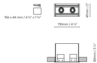
ANVIL LED MODULE R2
